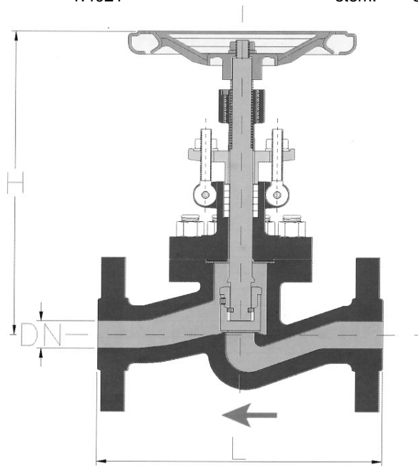
Type 017040
