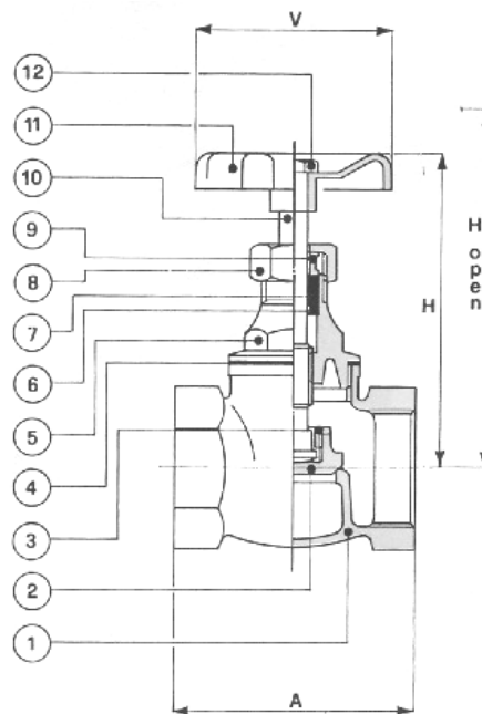
Type 032760 (metallisch dichtend/with metal seat) Type 033360 (mit PTFE-Dichtung/with PTFE-sealing)
